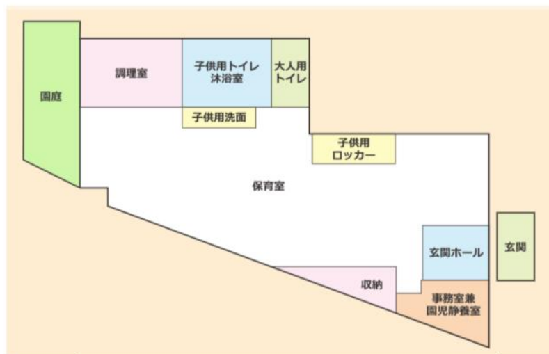
保育室①
